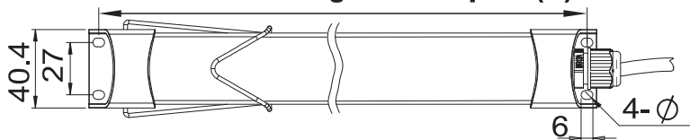
ねじ穴間の寸法 Mounting hole template(B)
